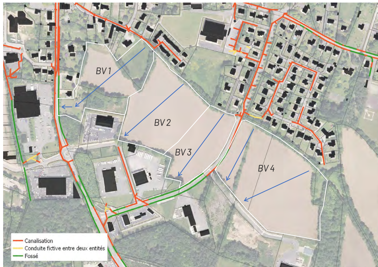
Document EOL : localisation et dimensionnement du réseau d'assainissement des eaux pluviales + bassins versants internes et sens des pentes
